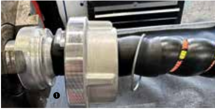
① Knaggenteil und den Sperring fest montieren ② Fertig eingebundene Seite mit der Kunststoffknickschutzspirale
